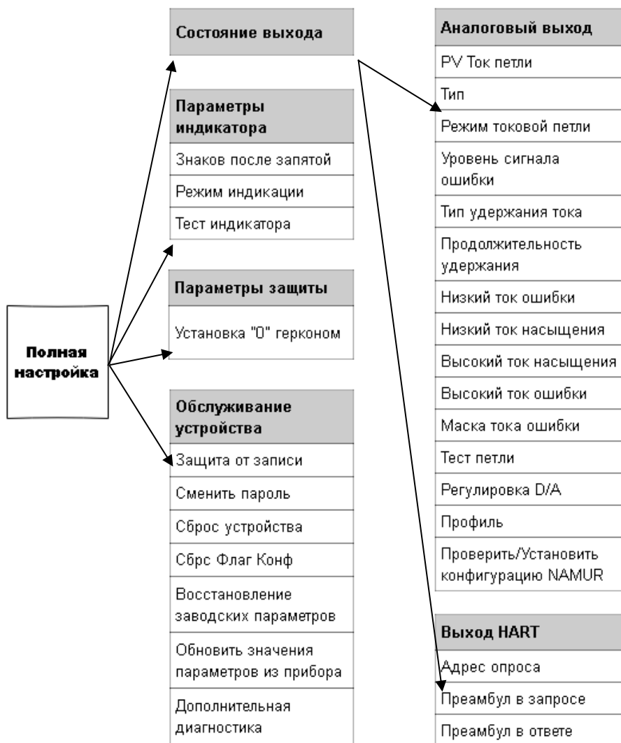
Рисунок Г.1 - Структура меню «В Сети» программы HARTmanager («Вид»/«В сети»), полевого коммуникатора или другого хост-устройства
